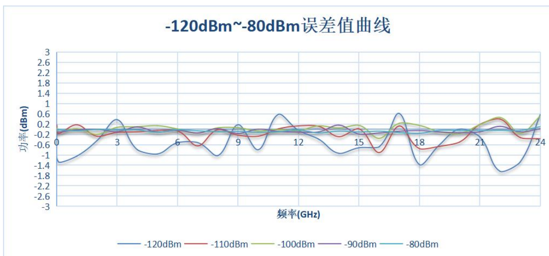
-120dBm~-80dBm 误差值曲线
