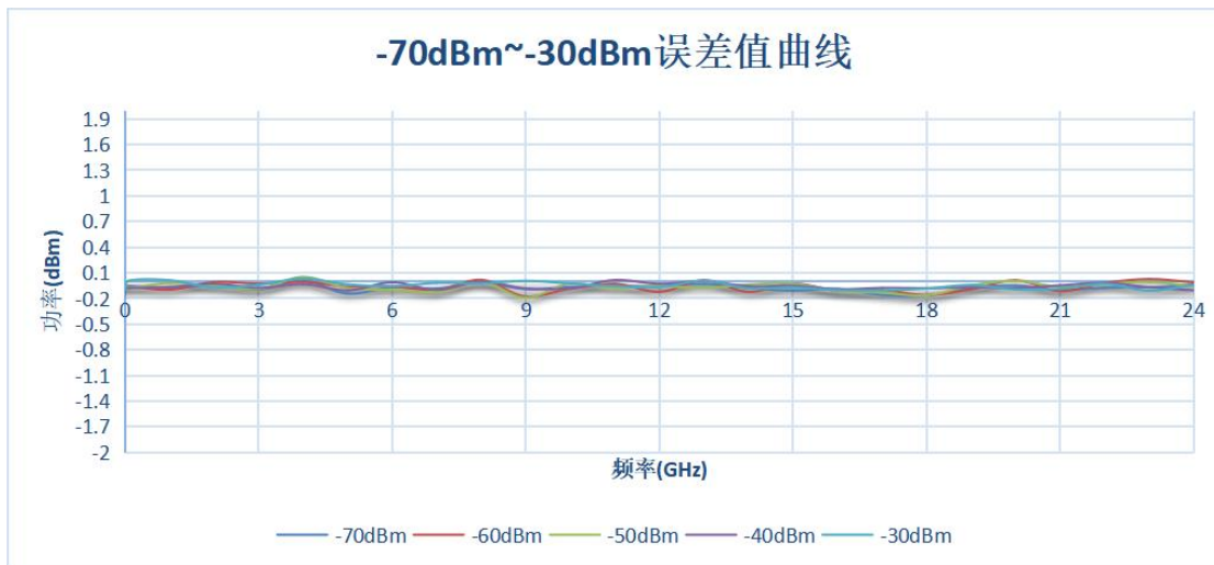
-70dBm~-30dBm 误差值曲线
