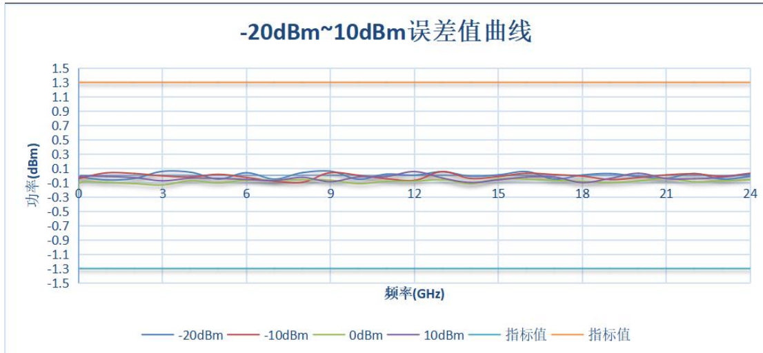
-20dBm~10dBm 误差值曲线
