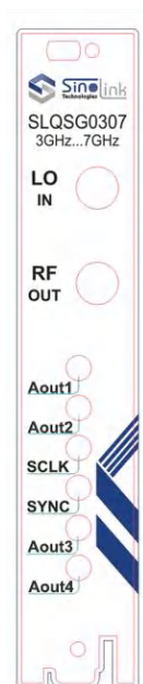
图 1 SLQSG0307 前面板
