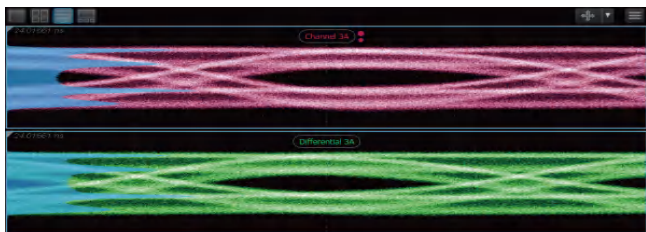
PPG码型发生器输出25.78125Gbps 注入DMI差模噪声示例
