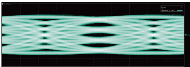
PPG码型发生器输出106.25Gbps PAM4眼图示例
