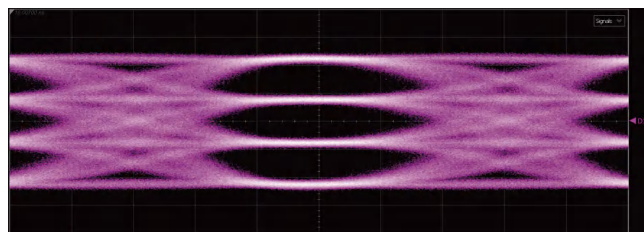
PPG码型发生器输出53.125Gbps 注入HFSJ 10MHz周期抖动示例
