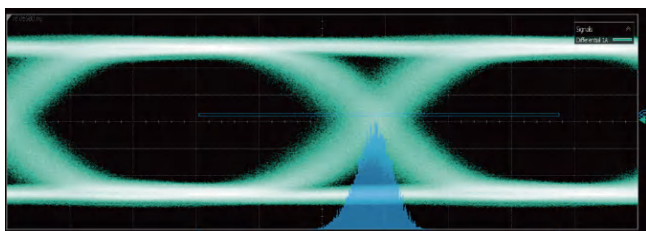
PPG码型发生器输出25.78125Gbps 注入RJ抖动示例
