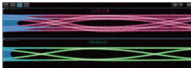
PPG码型发生器输出25.78125Gbps 注入CMI共模噪声示例
