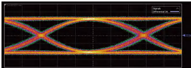
PPG码型发生器输出25.78125Gbps眼图示例
