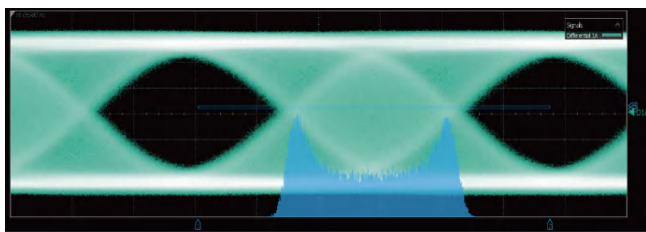
PPG码型发生器输出25.78125Gbps 注入HFSJ 10MHz周期抖动示例
