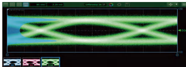
PPG码型发生器输出25.78125Gbps 注入BBN宽带白模噪声示例
